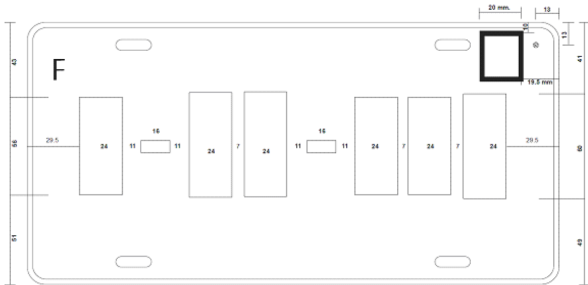
Figura 13 Para Vehículos de Demostración para las Entidades Federativas
