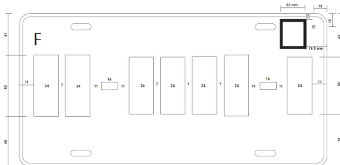
Figura 10 Para vehículos de corporaciones policíacas y de vigilancia Separación de caracteres (letras y dígitos), placas con siete caracteres y guiones. Acotaciones en milímetros. El ancho de los caracteres debe ser de acuerdo a lo indicado en la figura. Las dimensiones de los guiones serán de 16 x 5.6. Se incorporará la letra “T” y “F” según corresponda a la placa.
