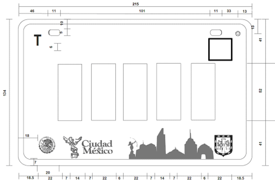
Figura 29 Privado motocicleta Ciudad de México y entidades federativas Separación de caracteres (letras y dígitos), placas con cinco caracteres. Acotaciones en milímetros. El ancho de los caracteres debe ser de acuerdo a lo indicado en la figura. Las dimensiones de los guiones serán de 16 x 5.6. Se incorporará la letra "T" y "F" según corresponda a la placa.
